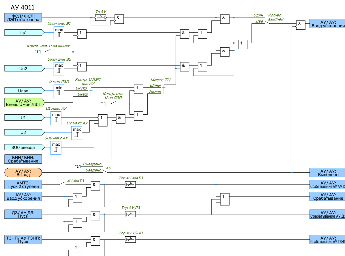
Рисунок 2.59 – Функциональная схема АУ
