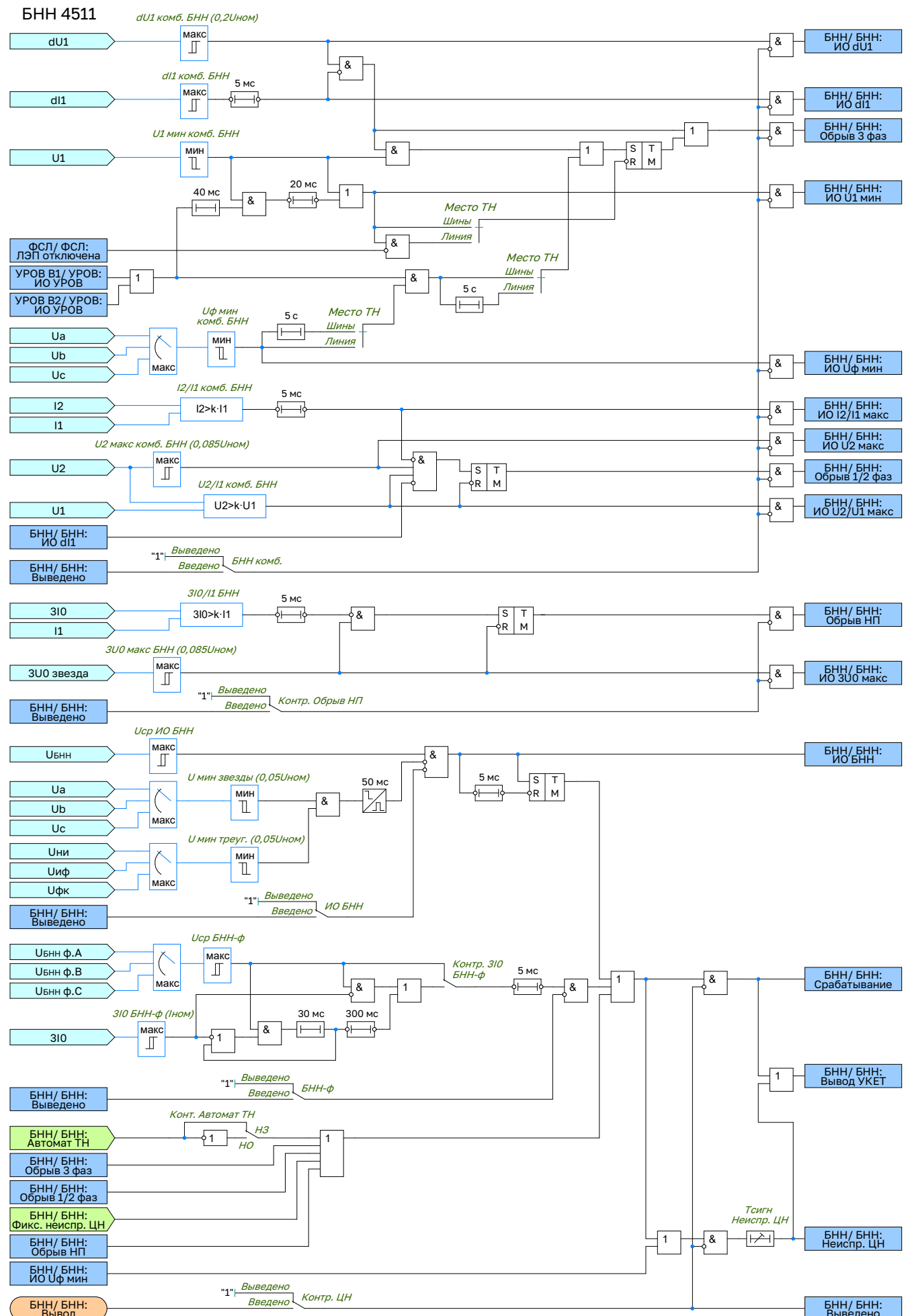
Рисунок 2.58 – Функциональная схема БНН
