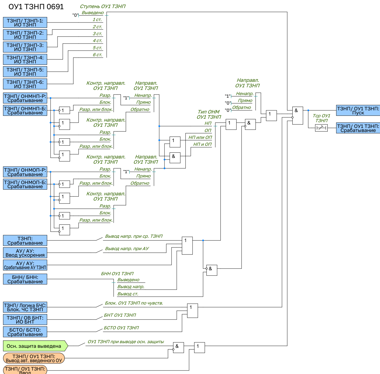
Рисунок 2.49 – Функциональная схема ОУ ТЗНП
