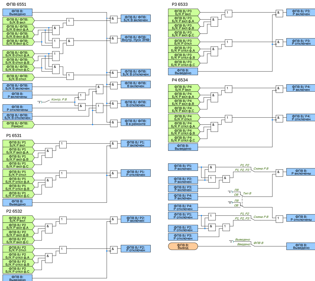
Рисунок 2.83 – Функциональная схема логики ФПВ В2
