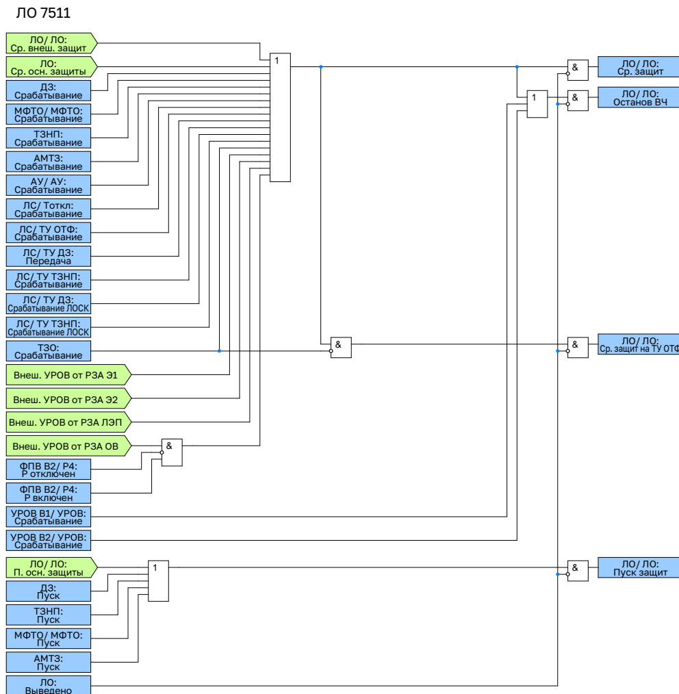
Рисунок 2.78 – Функциональная схема общей логики отключения
