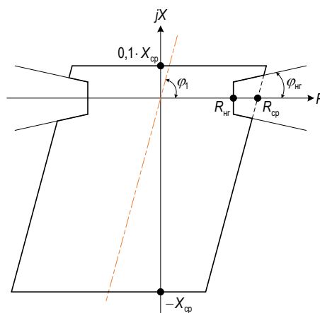
Рисунок 2.10 – Характеристика срабатывания блокирующего РС НВЧ3
