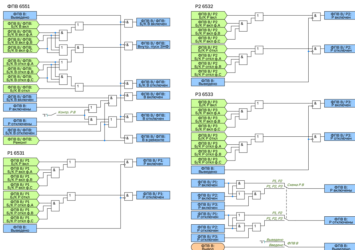
Рисунок 2.82 – Функциональная схема логики ФПВ В1
