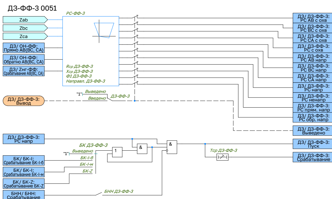
Рисунок 2.34 – Функциональная схема логики ДЗ-ФФ-3
