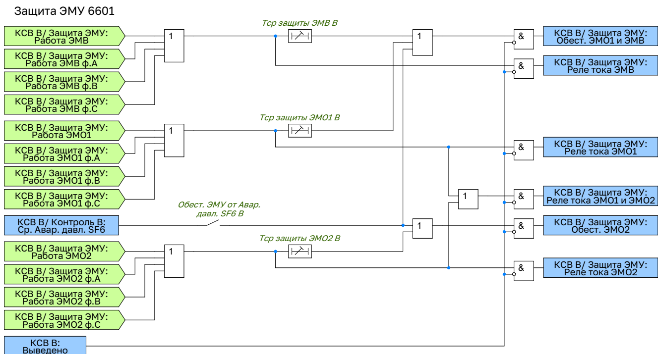
Рисунок 2.75 – Функциональная схема логики защиты ЭМУ выключателя
