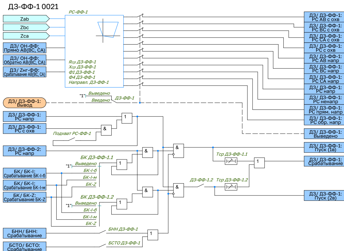
Рисунок 2.32 – Функциональная схема логики ДЗ-ФФ-1
